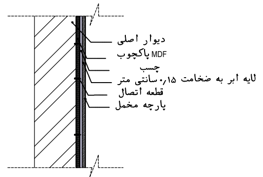
مقطع دیوار لمسه کوبی SC 1:5
