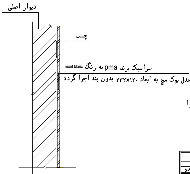
نحوه اتصال سرامیک به دیوار
