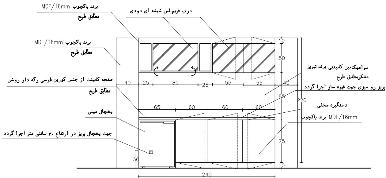
نما کابینت های فضای پذیرایی
