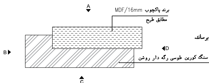
پلان کانتر پذیری
