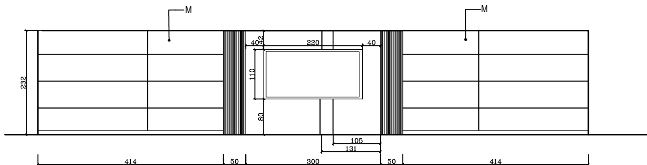
VIEW-D SC 1:20
